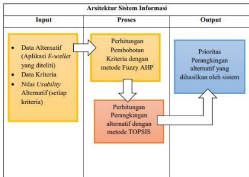
Gambar 3 Kerangka Arsitektur Sistem Uji Usability
