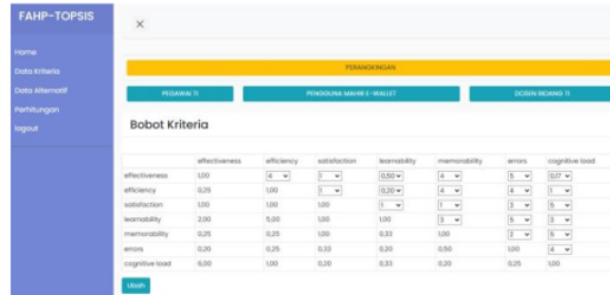
Gambar 6. Penentuan bobo oleh 3 responden ahli
