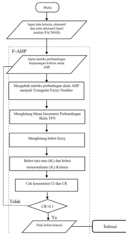
Gambar 7. Flowchart algoritma F-AHP pembobotan
