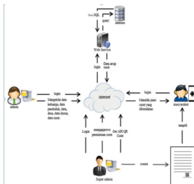
Gambar 3. Arsitektur sistem
